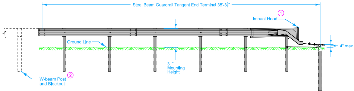
ELEVATION
